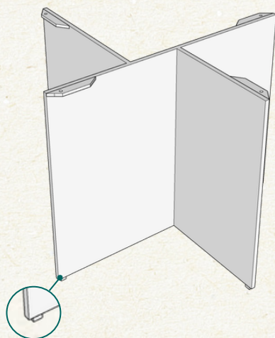
Detalhe da Sapata
